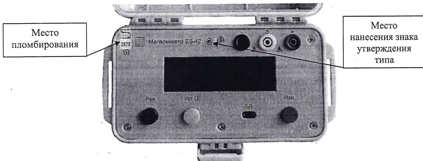
Рисунок 5 – Общий вид мегаомметров Е6-42
