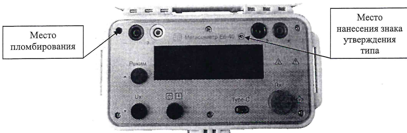
Рисунок 3 – Общий вид мегаомметров Е6-40 (горизонтальное исполнение корпуса)
