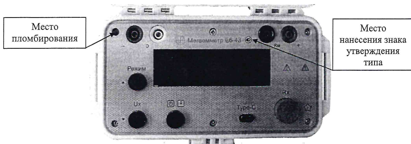
Рисунок 6 – Общий вид мегаомметров Е6-43
