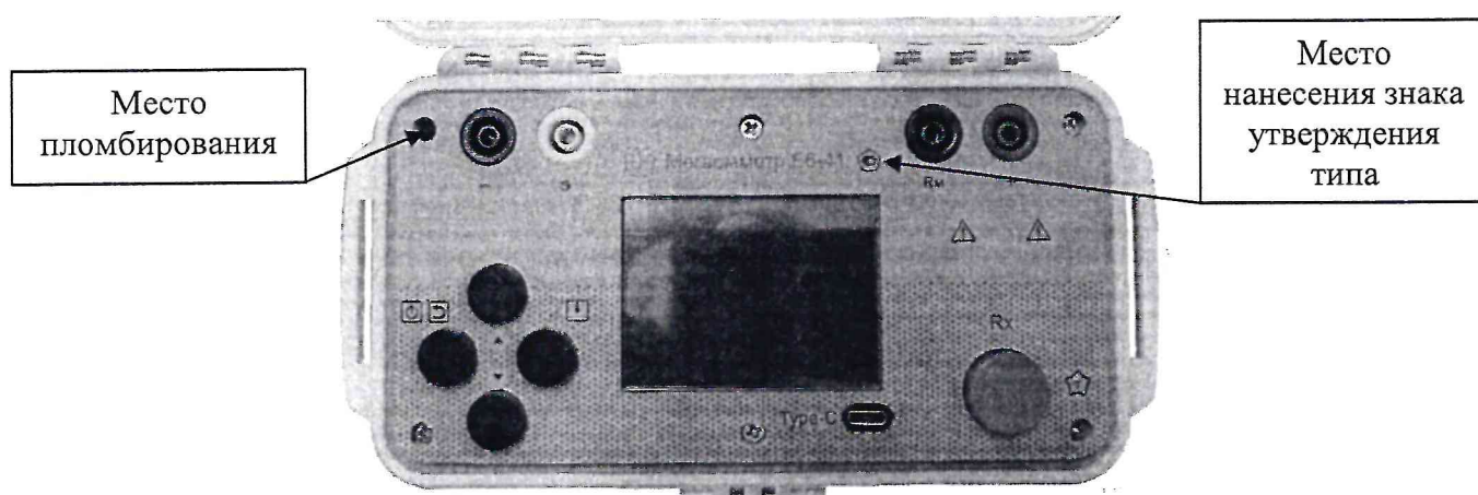
Рисунок 4 – Общий вид мегаомметров Е6-41 (горизонтальное исполнение корпуса)
