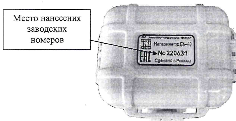
Рисунок 7 – Обозначение места нанесения заводских номеров на мегаомметры Е6-40, Е6-41 (вертикальное исполнение корпуса)
